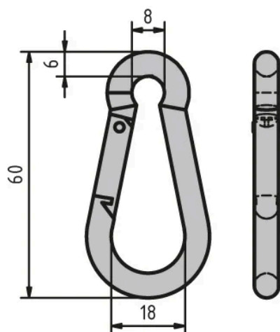
Karabinerhaken
